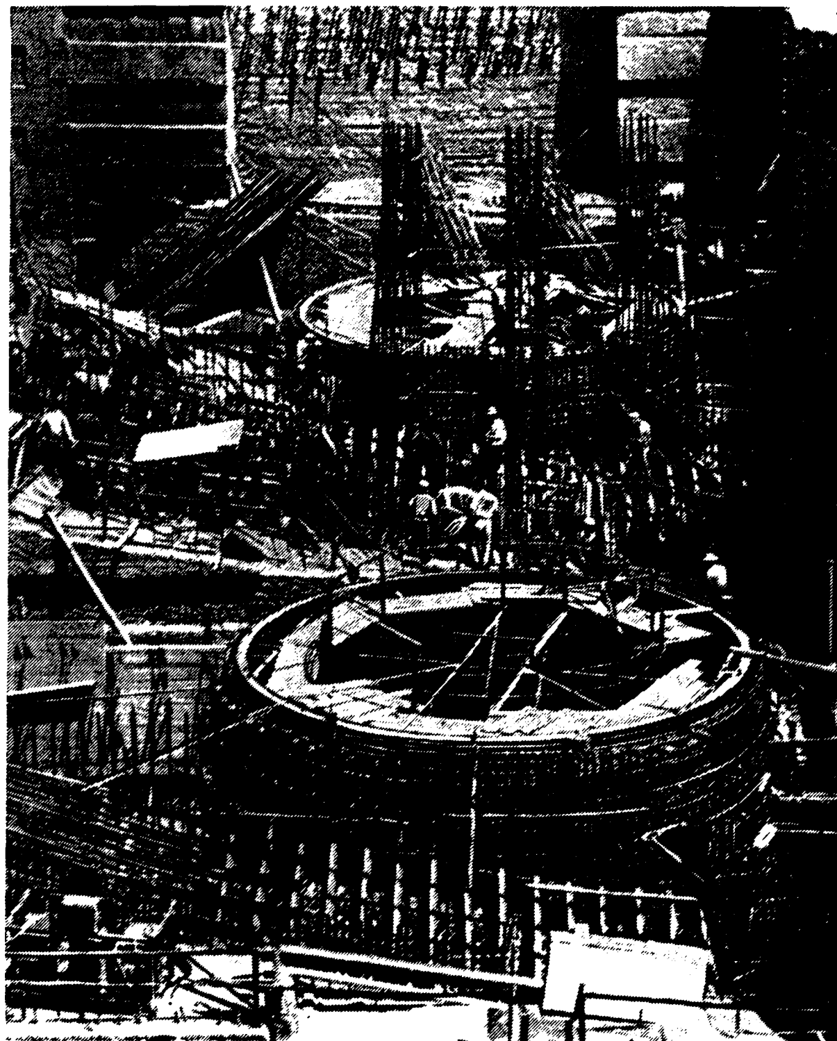
Монтаж Большой Асуанской ГЭС. 2-я очередь. Март 1966.
